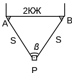
Рис. 11. Подвійний стінний знак
