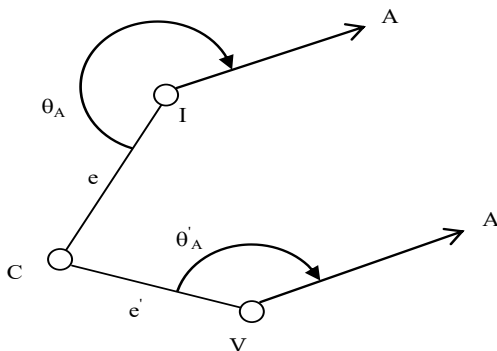
Рис.9. Елементи центрування та редукції
