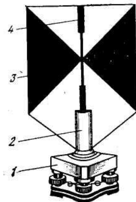
Рис.5. Візирна марка
