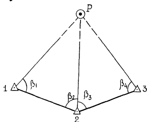
Рис.10. Пряма куттова засічка
